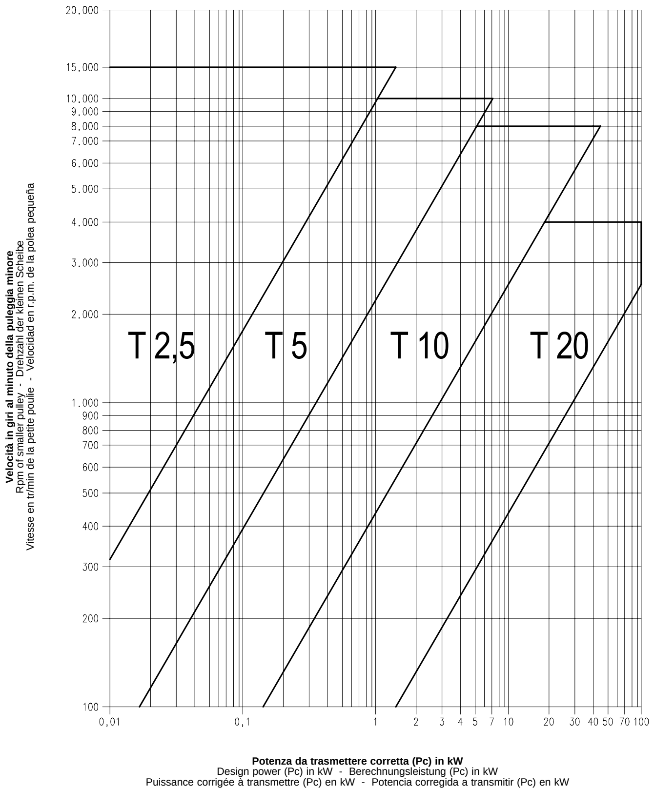
GRAFICO N. 1 - Per la scelta del passo della cinghia T TABLE Nr. 1 - T belt pitch selection DIAGRAMM Nr. 1 - Zur Auswahl der T Riementeilung DIAGRAMME Nr. 1 - Pour le choix du pas de la courroie T DIAGRAMA Nro. 1 - Para la elección del paso de la correa T
