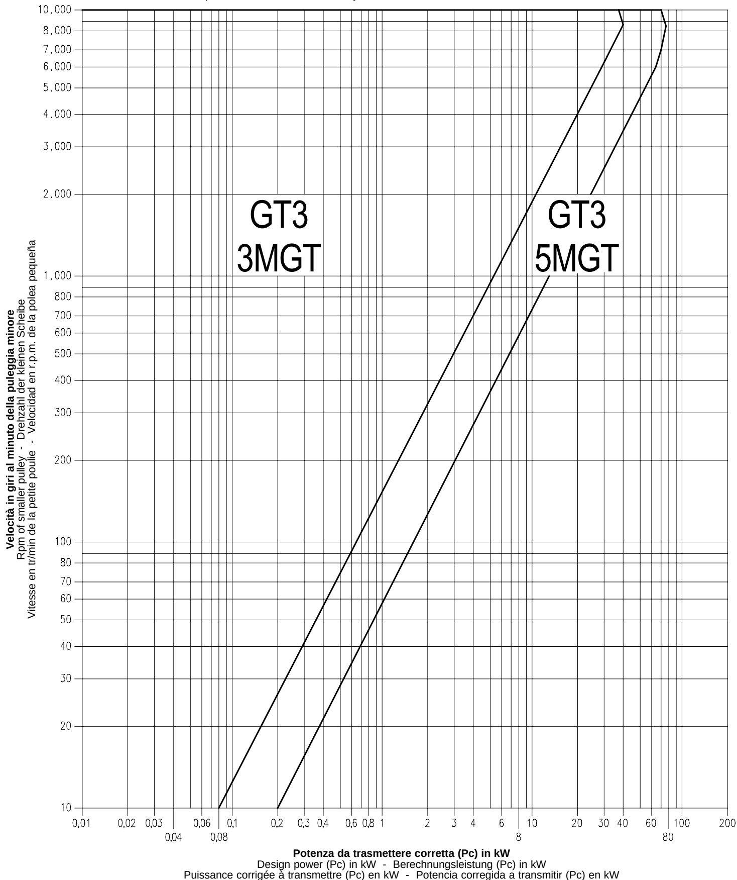
GRAFICO N. 5 - Per la scelta del passo della cinghia GT3® 3MGT e 5MGT TABLE Nr. 5 - GT3® 3MGT and 5MGT belt pitch selection DIAGRAMM Nr. 5 - Zur Auswahl der GT3® 3MGT und 5MGT Riementeilung DIAGRAMME Nr. 5 - Pour le choix du pas de la courroie GT3® 3MGT et 5MGT DIAGRAMA Nro. 5 - Para la elección del paso de la correa GT3® 3MGT y 5MGT
