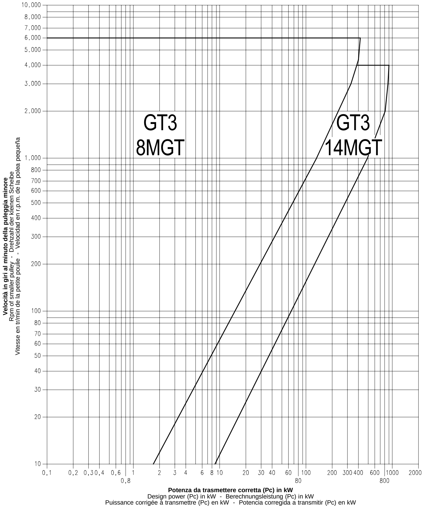
GRAFICO N. 6 - Per la scelta del passo della cinghia GT3® 8MGT e 14MGT TABLE Nr. 6 - GT3® 8MGT and 14MGT belt pitch selection DIAGRAMM Nr. 6 - Zur Auswahl der GT3® 8MGT und 14MGT Riementeilung DIAGRAMME Nr. 6 - Pour le choix du pas de la courroie GT3® 8MGT et 14MGT DIAGRAMA Nro. 6 - Para la elección del paso de la correa GT3® 8MGT y 14MGT
